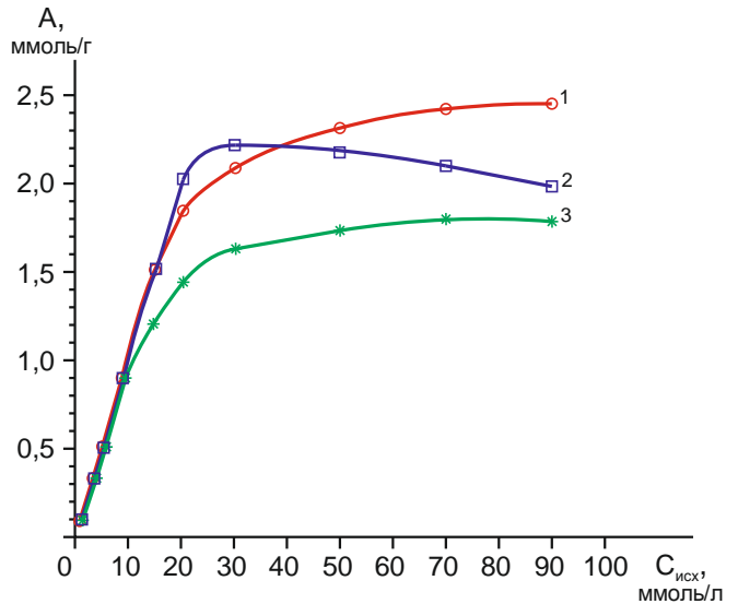
Рис. 19. Зависимости величин сорбционной ёмкости силикатно-кальциевых сорбентов от исходной концентрации катионов \text{Eu}^{3+} :
