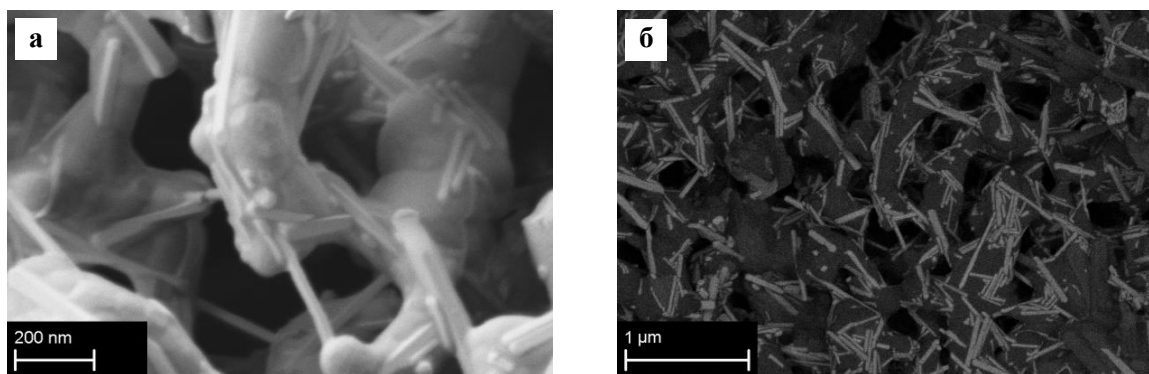
Рис. 22. РЭМ-изображение поверхности частиц композиционного материала на основе \text{CaSiO}_3 с нанесёнными наночастицами \text{Pr}_2\text{O}_3 и \text{Tb}_2\text{O}_3 (экстракционно-пиролитический метод получения) в режиме композиционного контраста (а) и топографического контраста (б)
