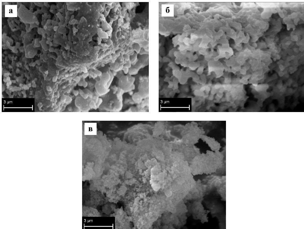
Рис. 4. РЭМ-изображение образцов силикатов кальция, полученных после обжига при температуре 950\text{ }^\circ\text{C} соответствующих гидросиликатов кальция (см. рис. 3)
